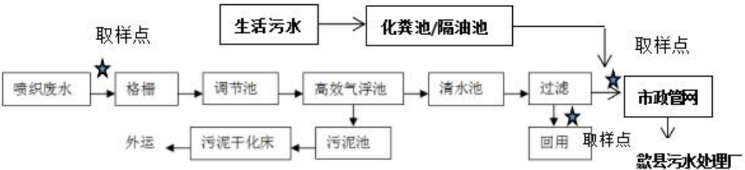
图 3-2 污水处理处理的工艺流程图及验收监测采样点示意图
