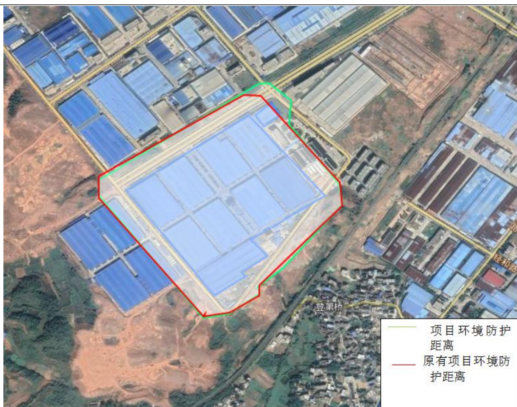
图 7-2 环境防护距离包络线图
