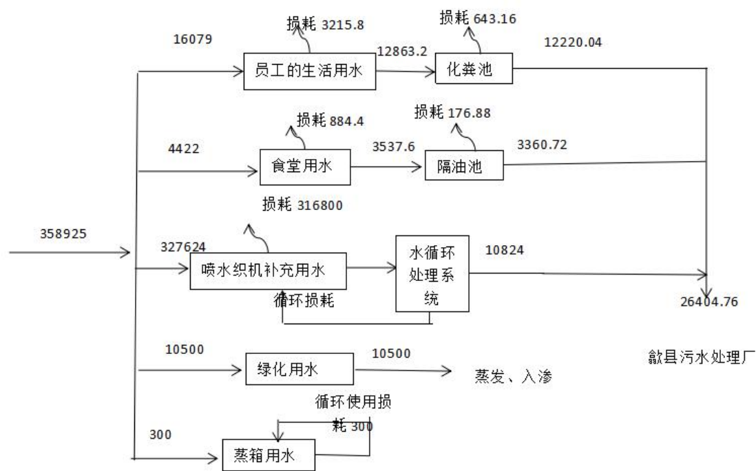
图 2-1 用排水平衡图（t/a）
